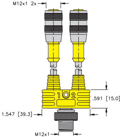
YBZ2-FSM 4.4/2FK 4(.4)T-*/*
